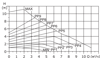
Рис. 12 Кривые режима управления пропорционального изменения давления.
