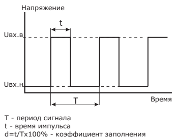
Рис. 16 Характеристики ШИМ-сигнала
