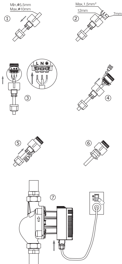
Рис. 8 Электроподключение
