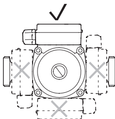
Рис. 4 Возможное положение клеммной коробки PROMO 15-9A, PROMO 15-12A
