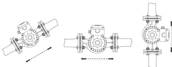
Рис. 59 Варианты монтажа
