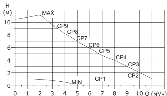
Рис. 43 Кривые режима управления с постоянным значением давления.
