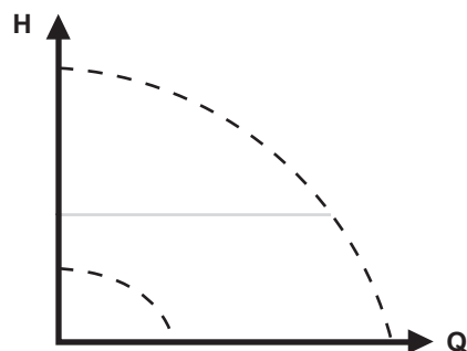
Рис. 57 Регулирование по постоянному давлению
